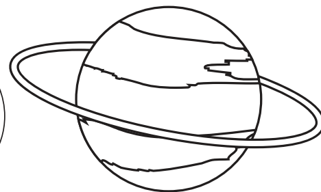
Uranus
